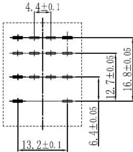
插座孔位图
